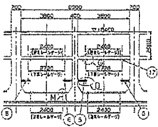
断面 B-B
